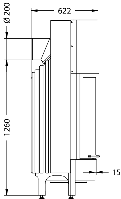
Seitenansicht M~1:20
