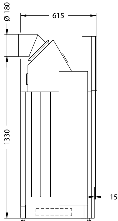
Seitenansicht M~1:20
