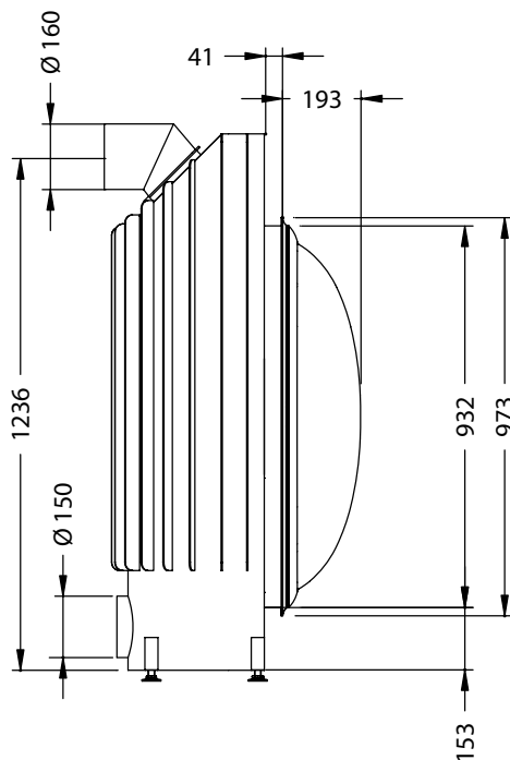
Seitenansicht M~1:20
