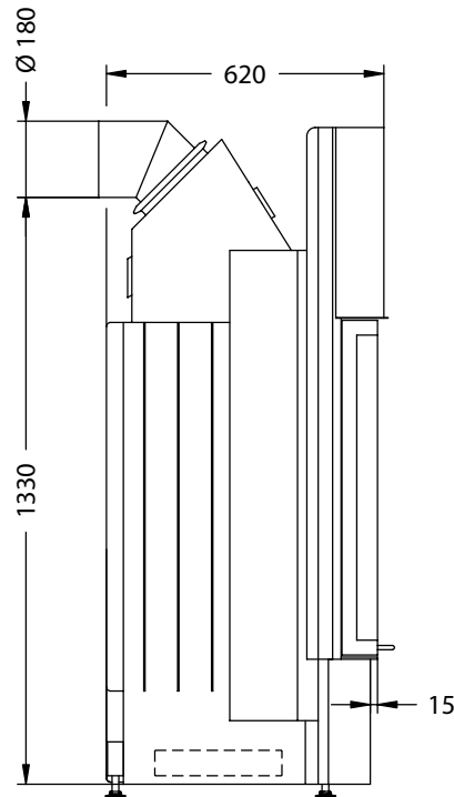
Seitenansicht M~1:20
