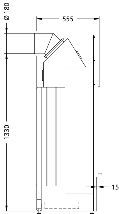
Seitenansicht M~1:20
