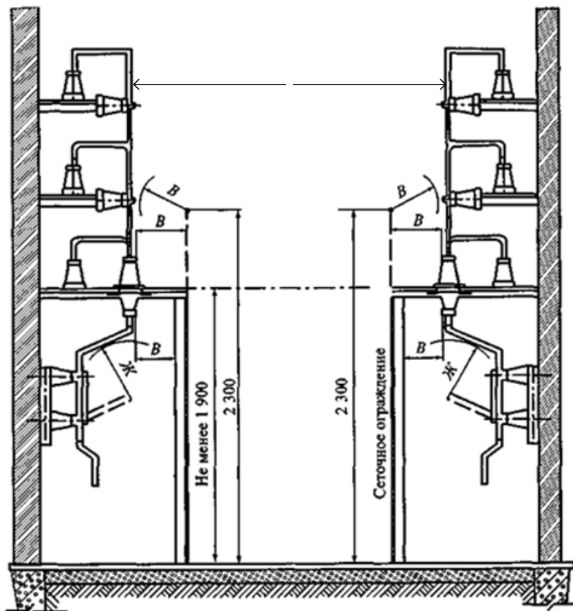
Рис. 6.2.16 – Наименьшие расстояния от неизолированных токоведущих частей в ЗРУ до сетчатых ограждений и между неогражденными неизолированными токоведущими частями разных цепей (таблица 6.2.9)
