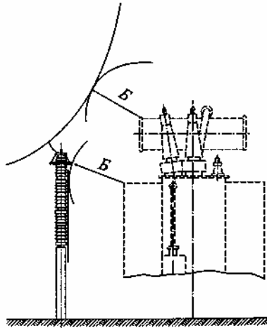
Рисунок 6.2.7 – Наименьшие расстояния от токоведущих частей до транспортируемого оборудования
