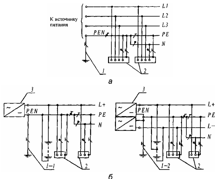
Рисунок 4.3.2. Подсистема TN-S переменного (а) и постоянного (б) тока
