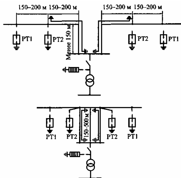
Рисунок 6.2.19 – Схемы защиты от грозовых перенапряжений ПС,присоединенных к ВЛ с помощью заходов длиной до 150 и более 150 м
