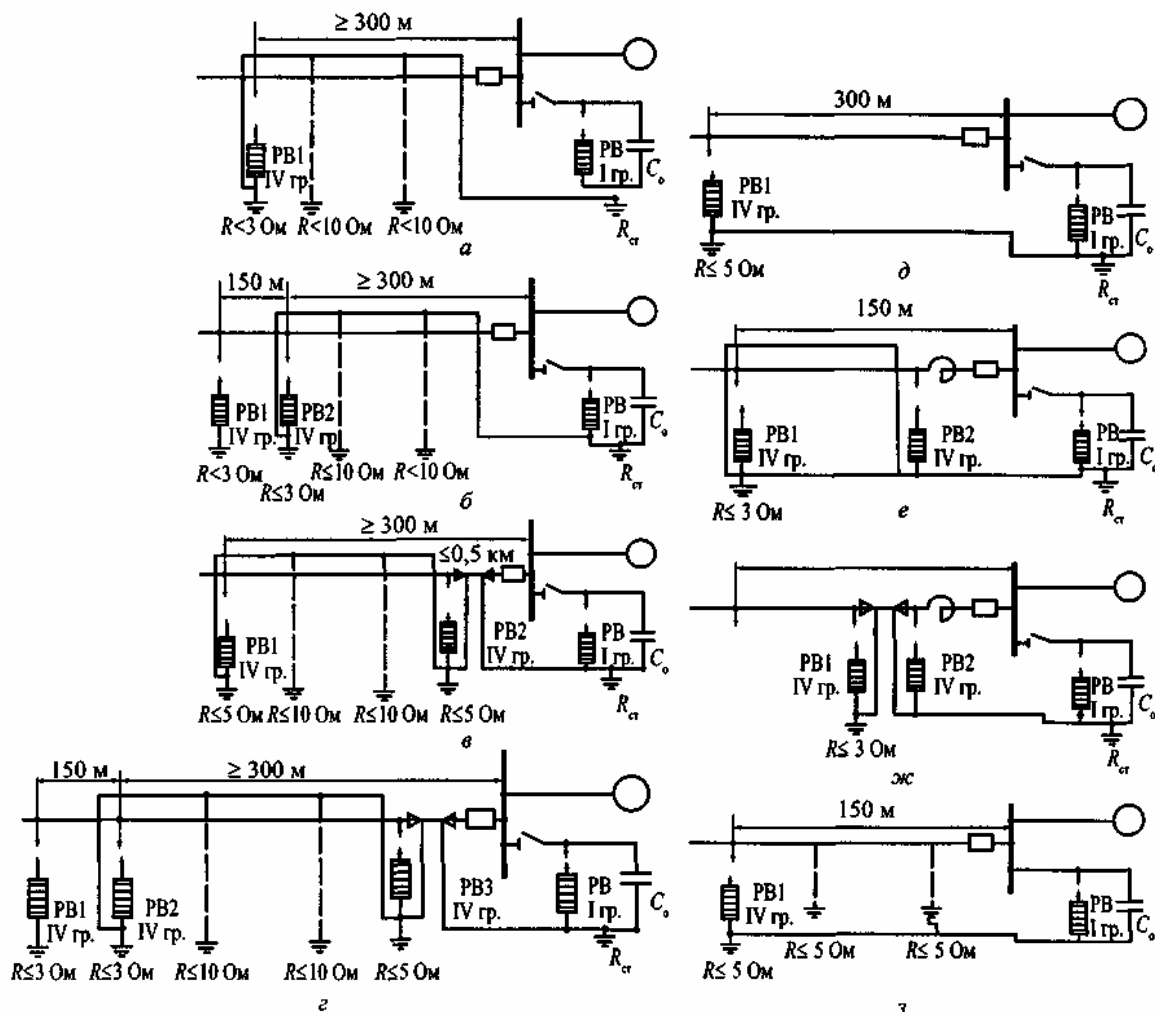
Рисунок 6.2.20 – Схемы защиты вращающихся электрических машин от грозовых перенапряжений
