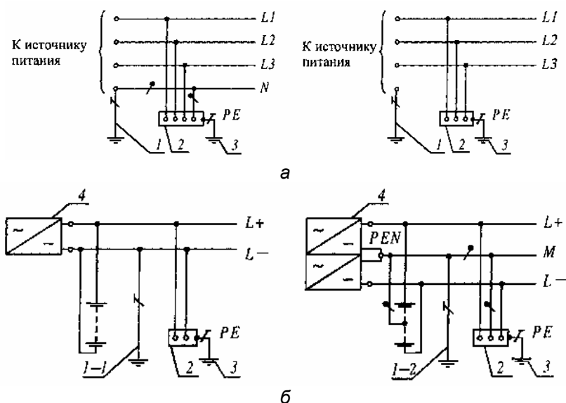
Рисунок 4.3.4 – Система IT переменного (а) и постоянного (б) тока
