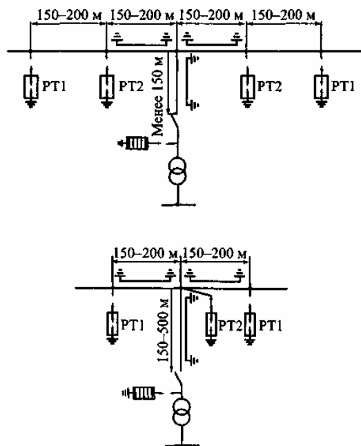
Рисунок 6.2.18 – Схемы защиты от грозовых перенапряжений ПС,присоединенных к ВЛ ответвлениями длиной до 150 и более 150 м
