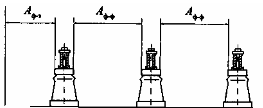
Рисунок 6.2.14 – Наименьшие расстояния в свету между неизолированными токоведущими частями разных фаз в ЗРУ и между ними и заземленными частями (таблица 6.2.9)
