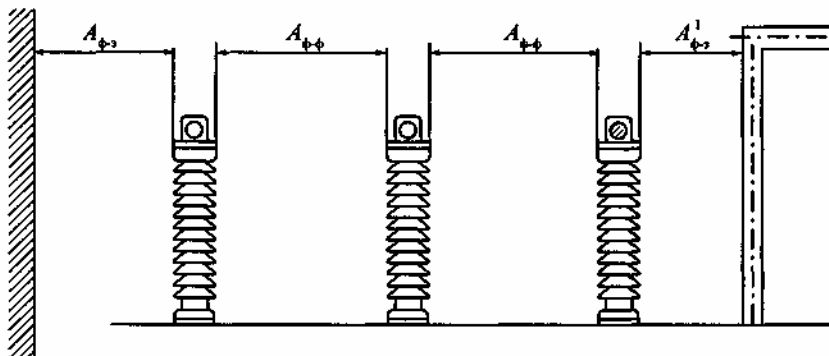
Рисунок 6.2.3 – Наименьшие расстояния в свету при жестких шинах между токоведущими и заземленными частями ( A_{ф-з} , \dot{A}_{б-ф}^1 ) и между токоведущими частями разных фаз ( A_{ф-ф} )
