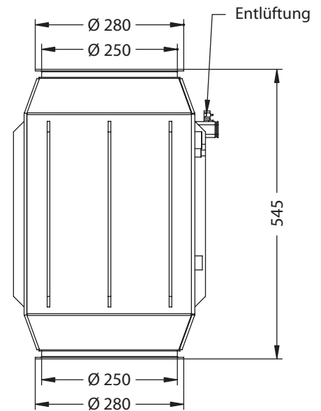
Seitenansicht M~1:10
