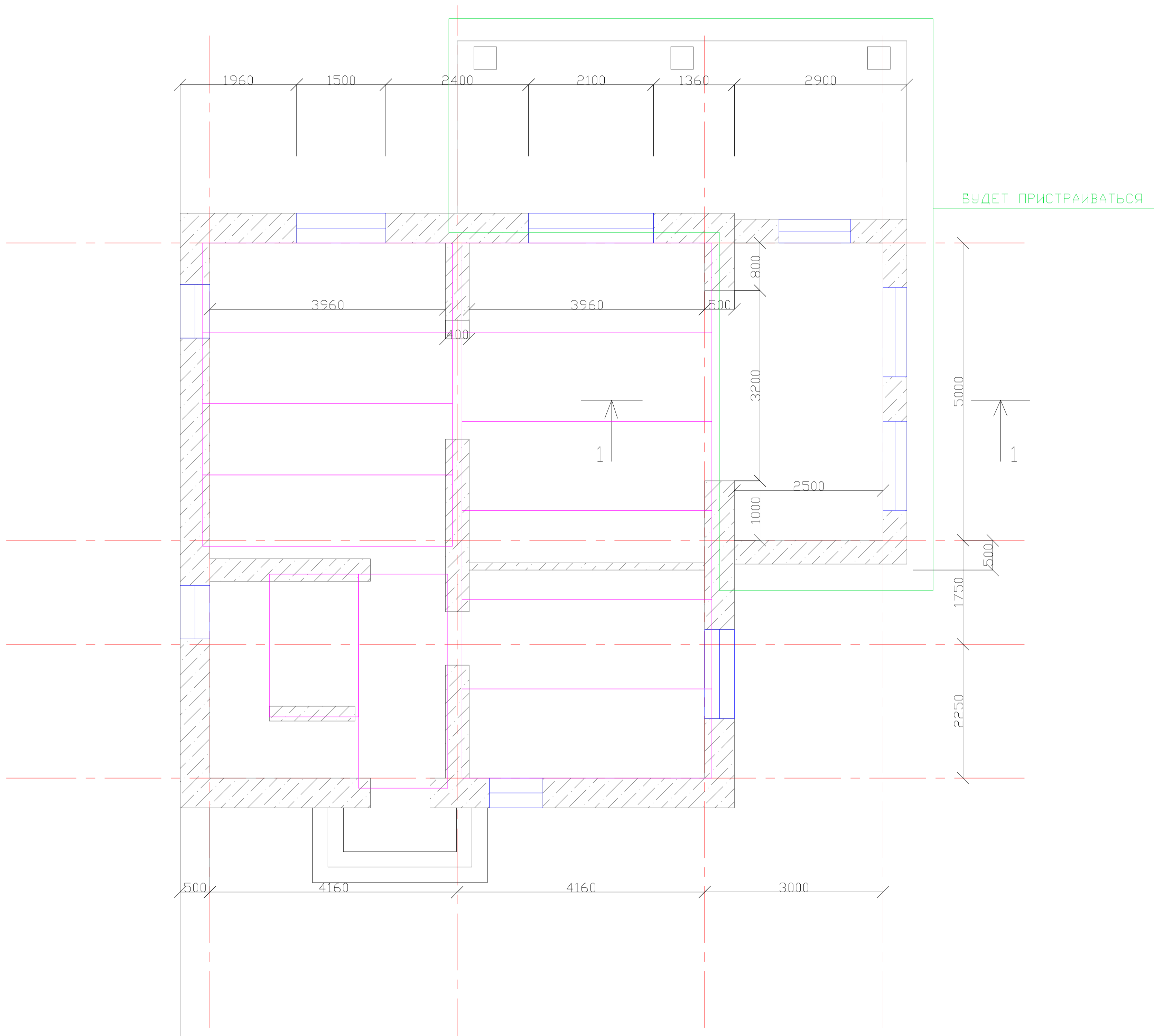
План несущих стен с укладкой плит перекрытия
