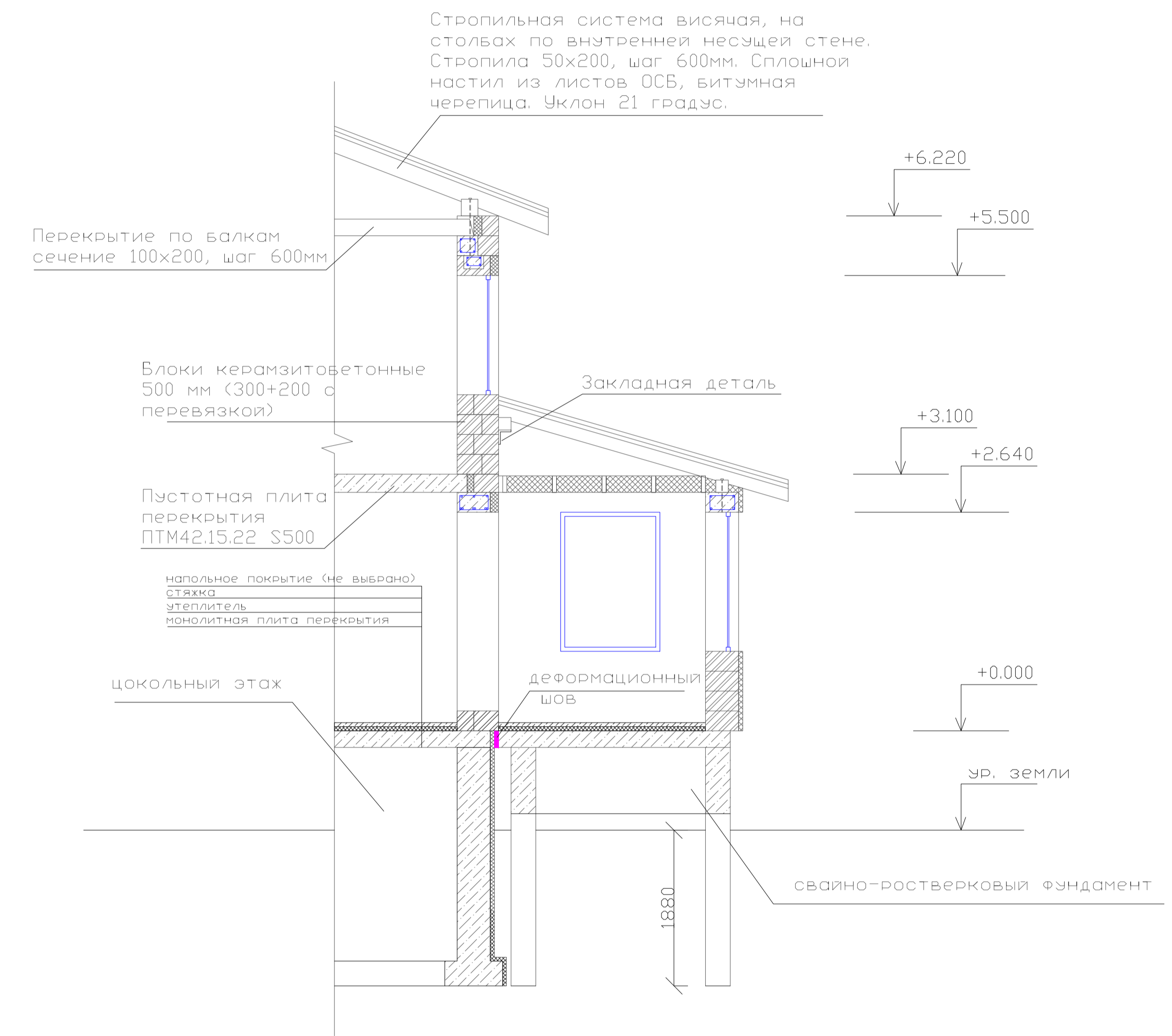
Разрез 1-1
