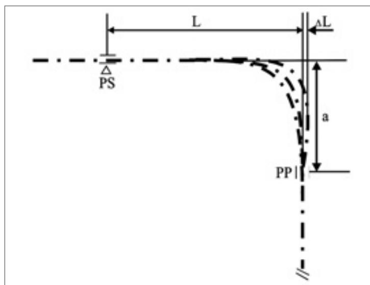
Рис. 49. Самокомпенсация труб PE-RT, PE-Xc, PE-RT/Al/PE-HD.
