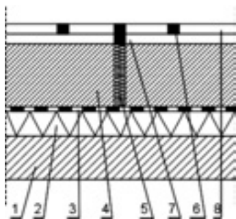
Рис. 134. Конструкция пола, покрытого керамической плиткой, с разделительным швом.
