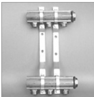
Рис. 36. Распределитель с ниппелями для конусных соединителей (серия 61).
