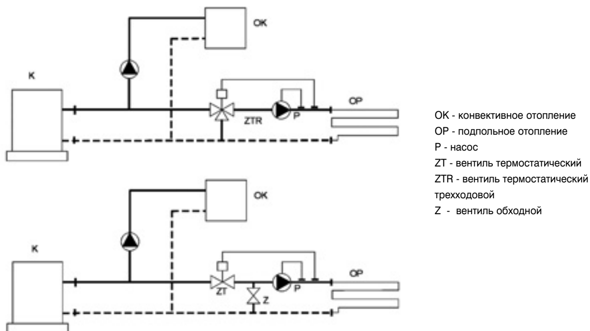
Рис.145. Смесительные системы, понижающие параметры теплоносителя.
