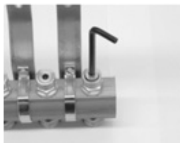
Рис. 154b. Способ выполнения предварительной настройки на запорно - регулирующем вентиле, вмонтированном на обратном коллекторе распределителя.
