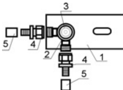
Рис. 234. УЗЕЛ «PPO-SR18k» - одна водоразборная точка с ответвлением (угловым) на холодную или горячую воду к последующей водоразборной точке.
