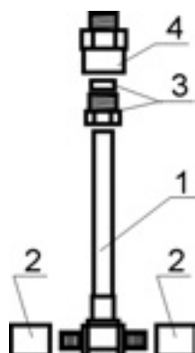
Рис. 236. УЗЕЛ «PPO-ZT18» «PPO-ZT25» - одна водоразборная точка холодной или горячей воды
