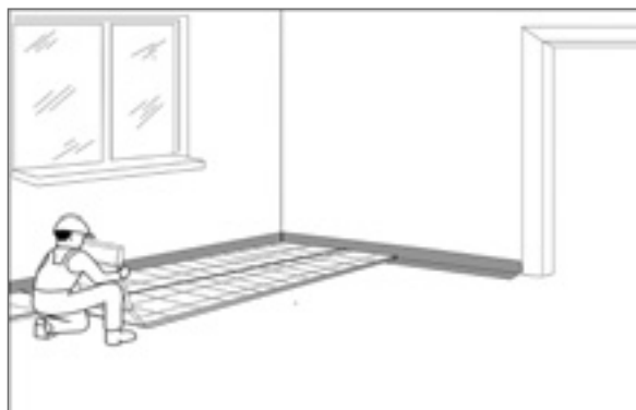
Рис. 141. Разложить пенополистирол с верхним слоем из ПЕ.
