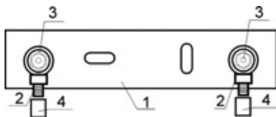
Рис. 237. УЗЕЛ «PPK-Z18» - две водоразборные точки конечные холодной и горячей воды.
