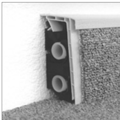
Рис. 95. Плинтус типа T.
