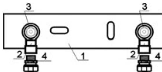
Рис. 238. УЗЕЛ «PPK-S18» «PPK-S25» - две водоразборные точки конечные холодной и горячей воды.
