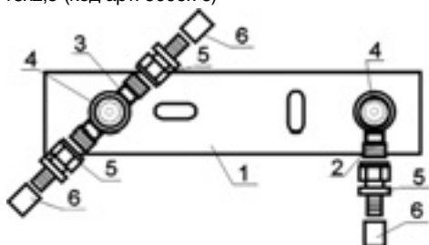
Рис. 253. УЗЕЛ «PPOZ-SR18pr» - две водоразборные точки с ответвлением (проходным) на горячую воду к последующей водоразборной точке.
