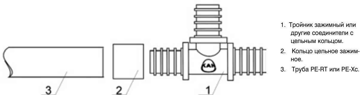
Рис. 14. Схема соединения с цельным кольцом, натягиваемым прессом.
