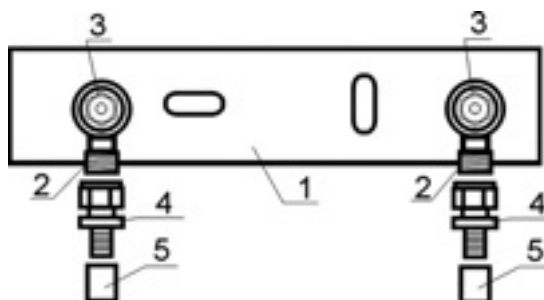
Рис. 239. УЗЕЛ «PPK-SR18» - две водоразборные точки конечные холодной и горячей воды.
