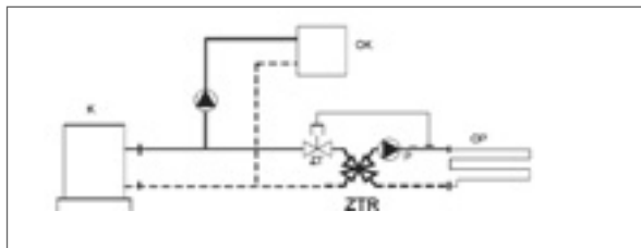
Рис. 146. Схема смесительной системы с полуавтоматическим регулированием:
