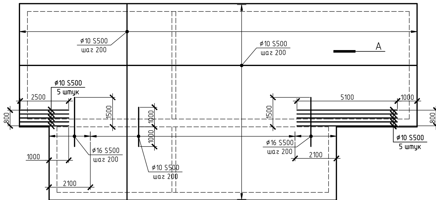
Схема раскладки нижней арматуры
