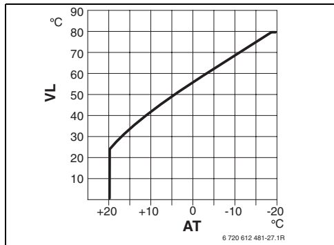
Рис 21 Основная настройка отопительной кривой для подогрева с использованием радиаторов
