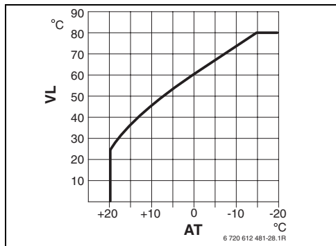
Рис 22 Основная настройка отопительной кривой для подогрева с использованием конвекторов
