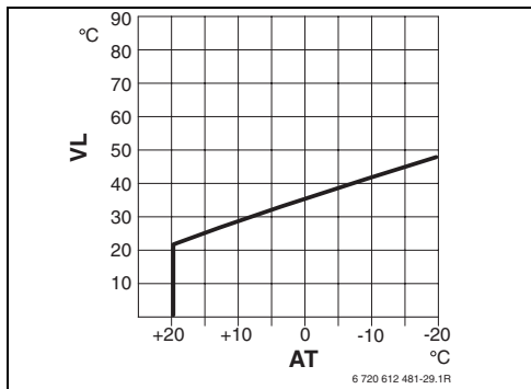
Рис 20 Основная настройка отопительной кривой для подогрева пола
